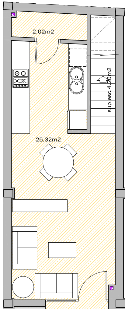
PLANTA BAJA
